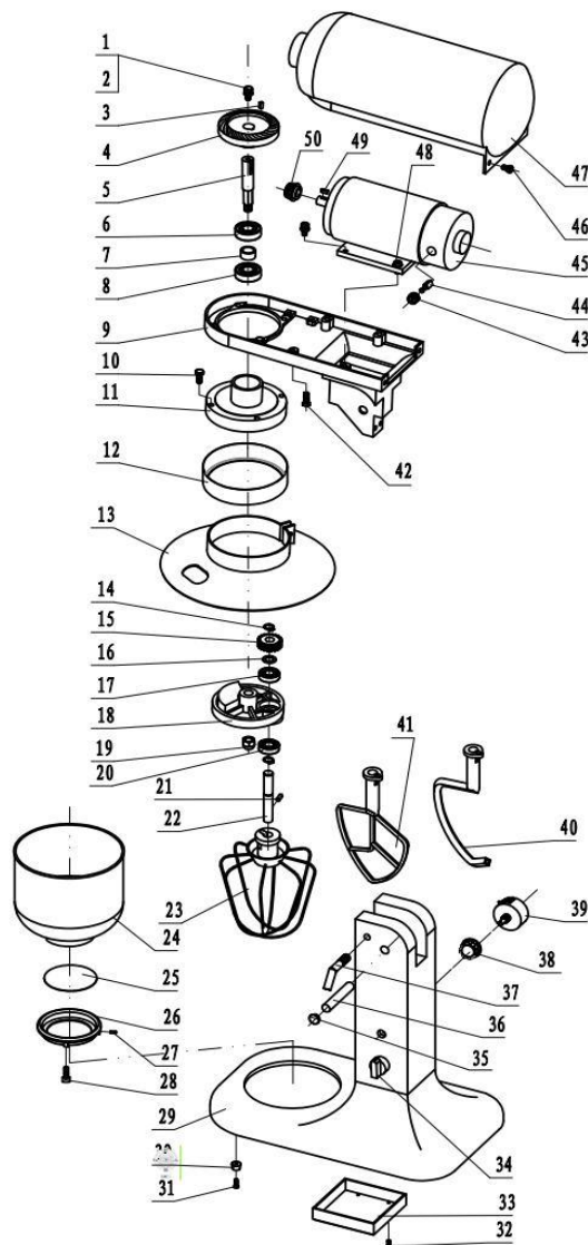
Рис. 1 Деталировка:
