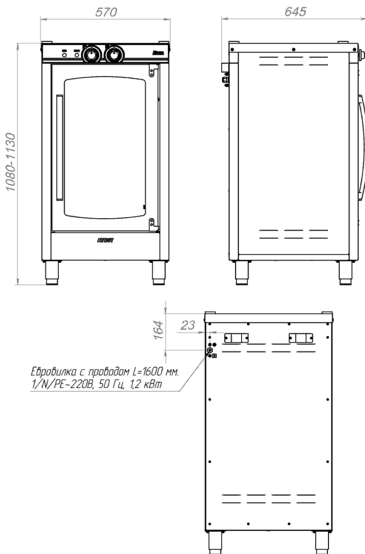
Рис.6. Общий вид и схема подключений ШП-10-430.330-01.
