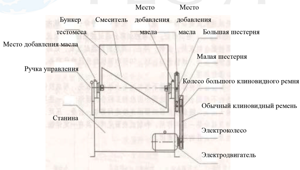
Схема конструкции машины HWY25
