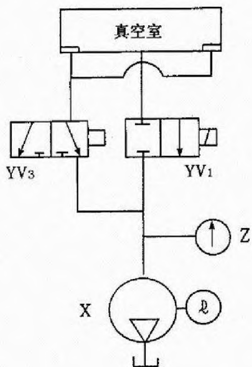
Однокамерный вакуумный запайщик с аэрацией
