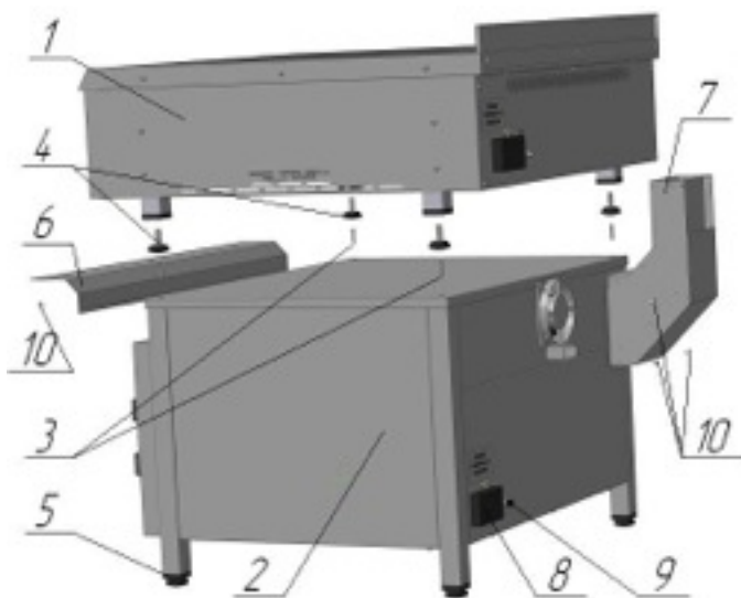
Рисунок 2: Схема установки плиты ПКИ-4ПР на шкаф духовой серии ПДЭ
