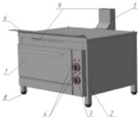
Рисунок 1.: Общий вид шкафа духового серии ПДЭ
