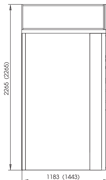
Вид А
